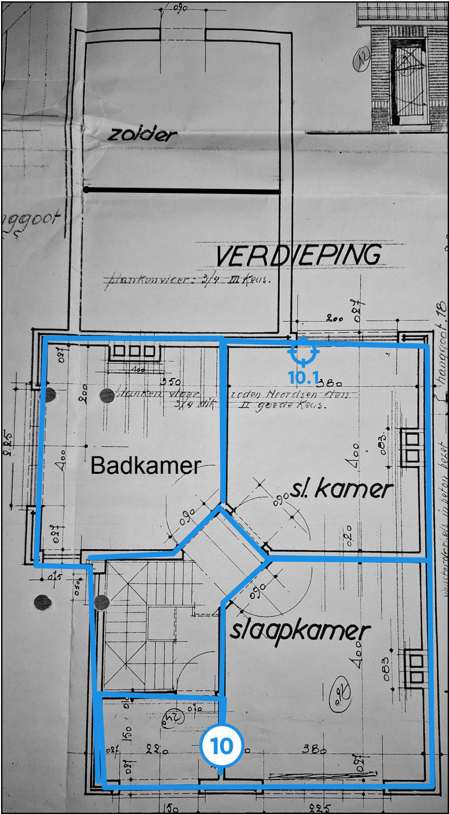
Legende van plan 1.7: Verdiep 1 deel 2
