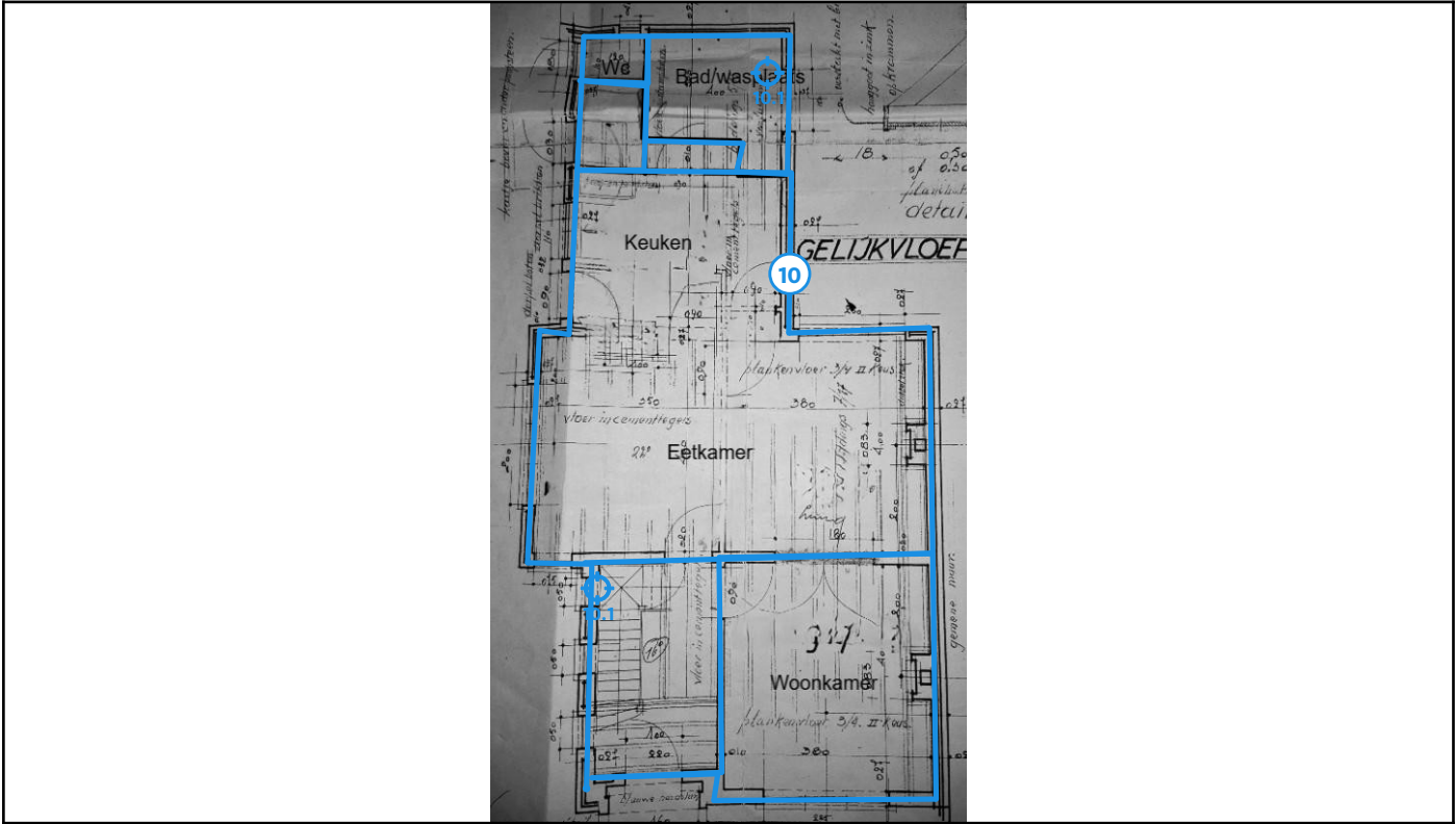
Legende van plan 1.3: GVL deel 1
